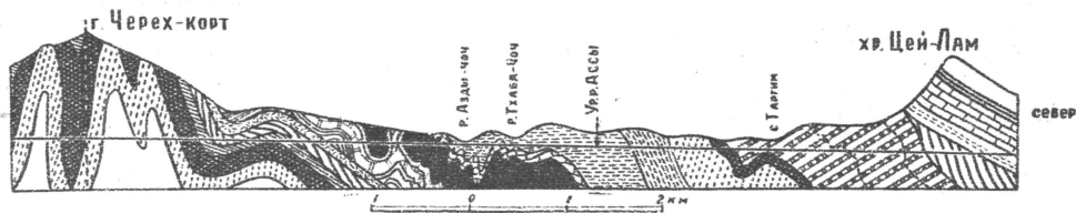
Характер залегания пород в северной части Кавказского хребта (разрез горы).
