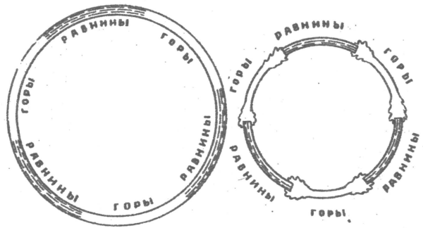
Начальная стадия охлаждения оболочки земного шара.
