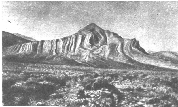
Гора в Пенсильвании. Морской известняк. Почти вертикальный пласт толщиной в 2000 футов.
