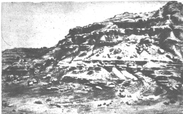
Горизонтальный «красный пласт», состоящий из наслоений красного песчаника и глинистого сланца. Северная Аризона.
